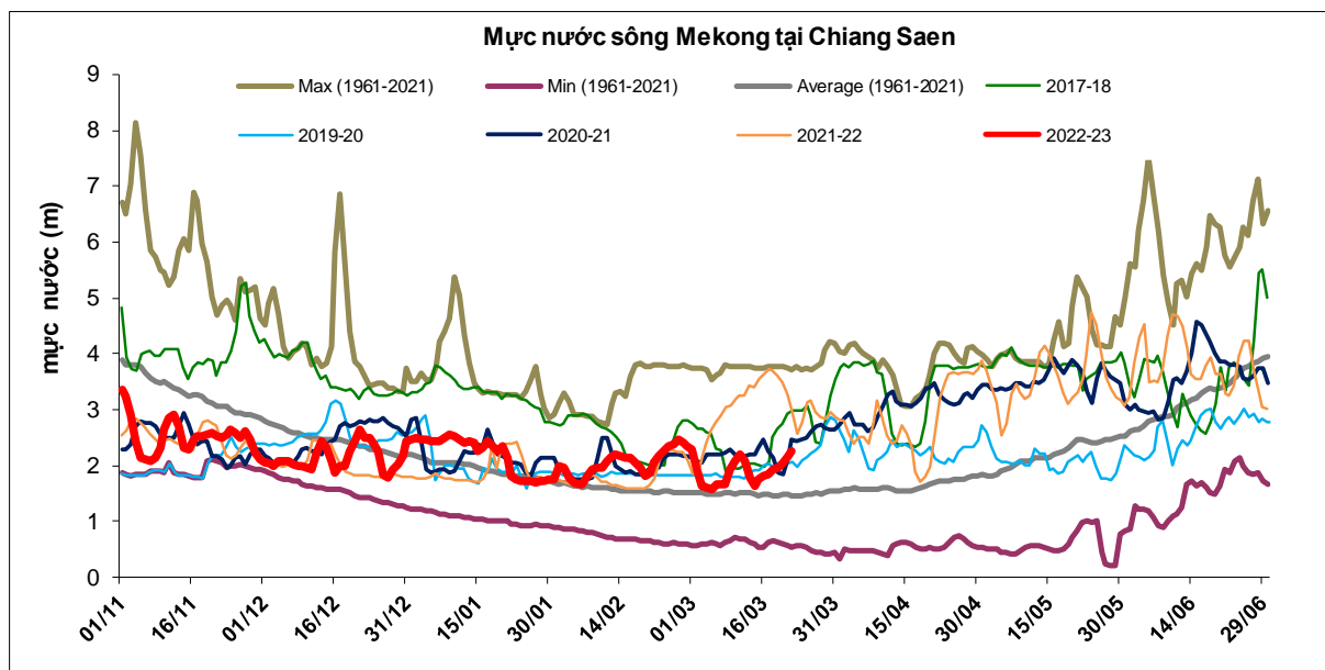
Hình 2. Diễn biến mực nước tại Chiang Saen –Thái Lan, cập nhật 22/3/2023
