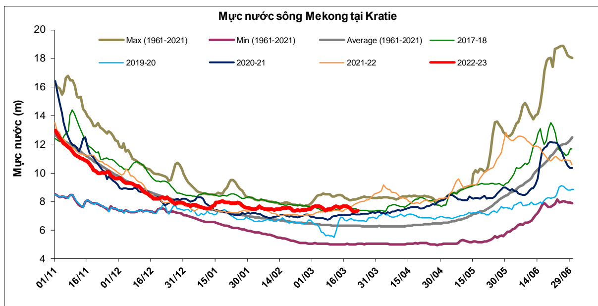
Hình 3. Diễn biến mực nước về qua trạm Kratie, cập nhật ngày 22/3/2023
