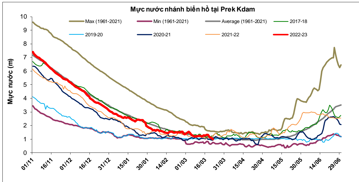
Hình 1. Diễn biến mực nước trạm Prek Kdam - Biển hồ, cập nhật ngày 22/3/2023
